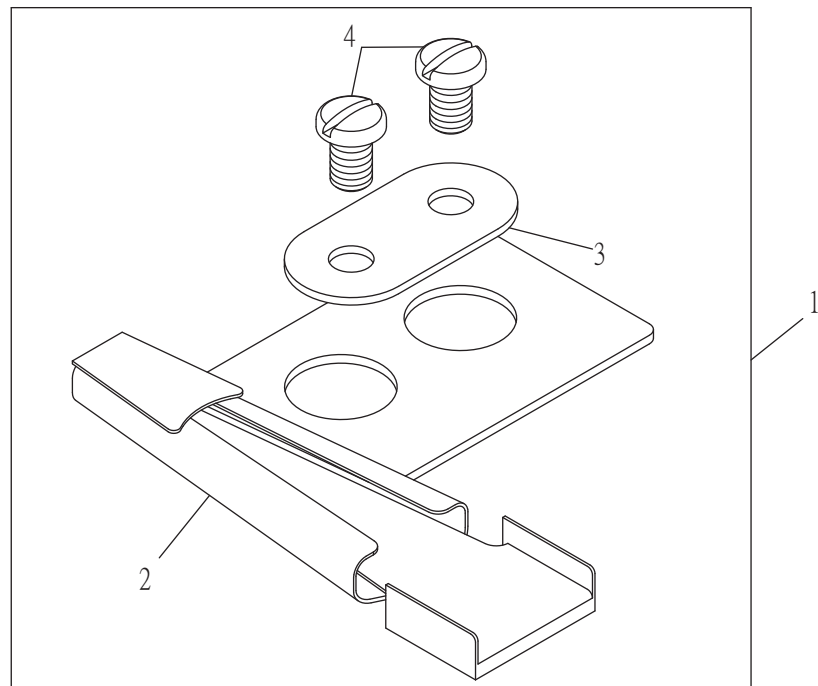
壓腳編號列表 Presser Foot
