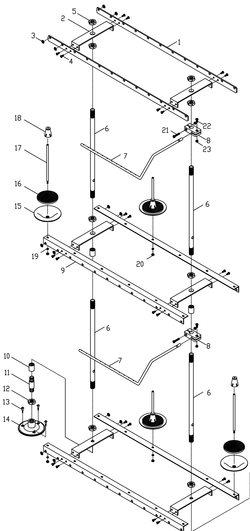
零件用量列表 Amt. Req.
