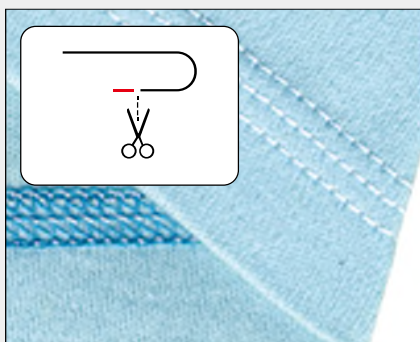
細筒型左切刀 Small Cylinder Left Trimmer CT98/ CTD98/ CTU98/ CXM28/ CXU28
