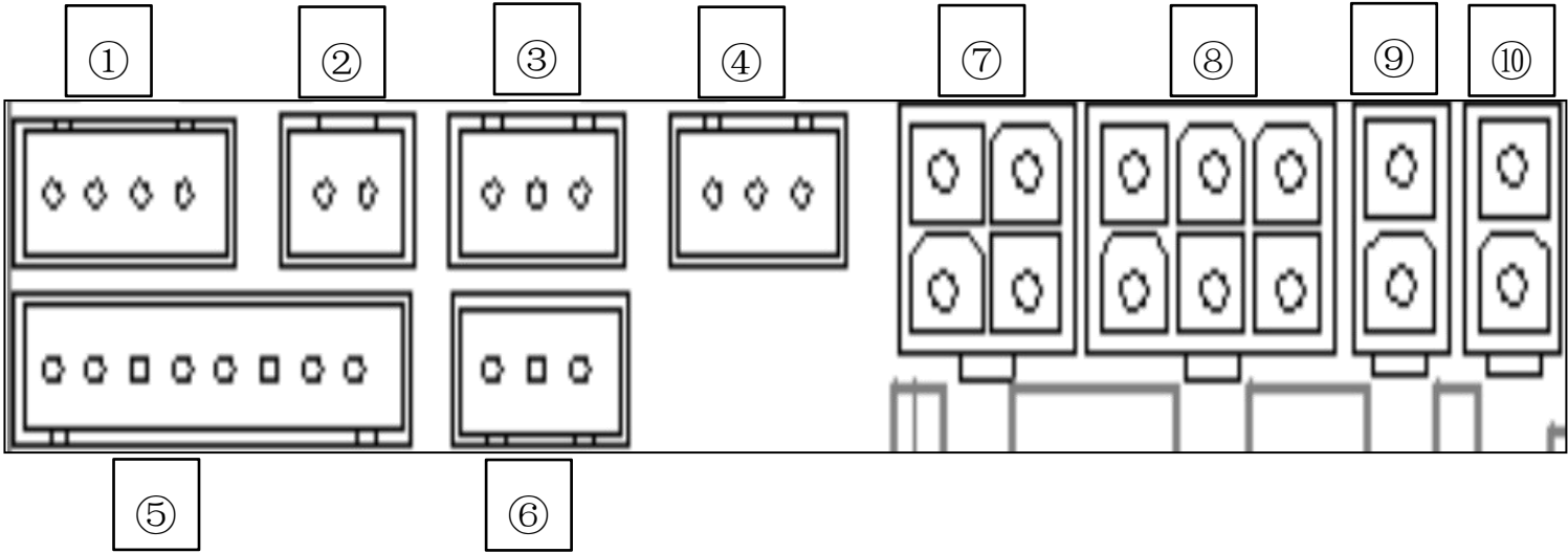
下光眼线端口 Down sensor wire port
