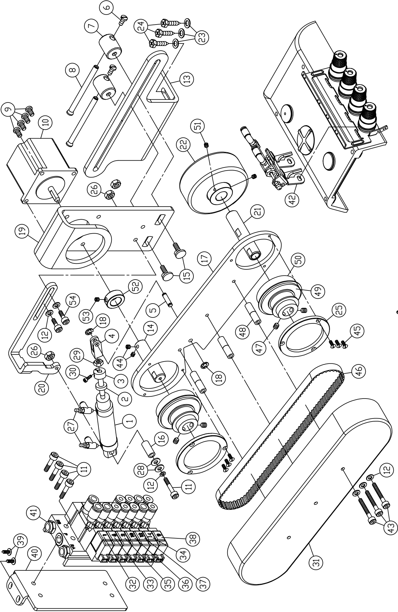
2.TR037(2) 擴張滾輪組零件列表 PARTS LIST FOR ROLLEER SET
